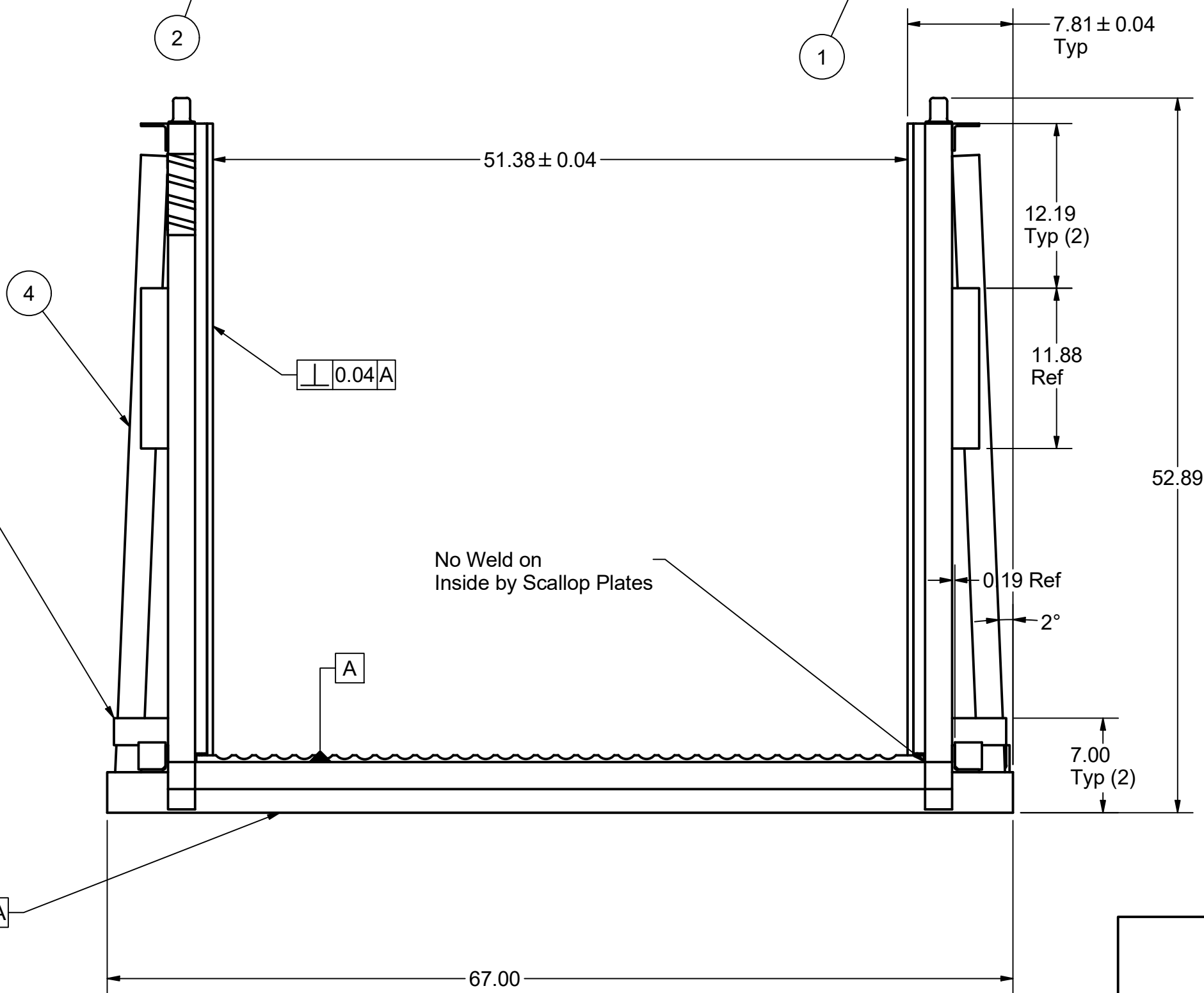
DETAIL A SCALE 0.22 : 1
